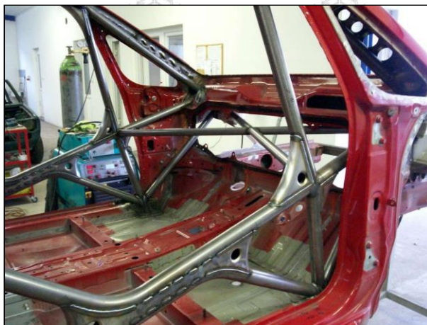
NAVIGÁTOR OLDALI VÁLL ÖV RÖGZÍTÉS SHOULDER HARNESS ATTACHMENT - CO-DRIVER
