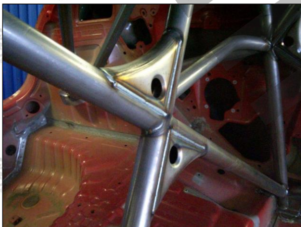
A BUKÓKETREC BEÉPÍTÉS UTÁN NEM LÁTHATÓ RÉSZEI NOT VISIBLE DETAILS OF CAGE
