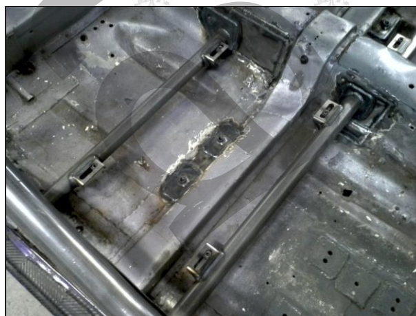
PHOTO 34 HEGESZTETT ÜLÉSTARTÓ WELDED SEAT MOUNTING
