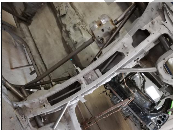
ELSŐ-/OLDALÍV RÖGZÍTÉSE AZ "A" OSZLOPHOZ FRONT ROLLBAR TO "A" PILLAR ATTACHMENT
