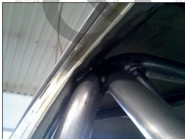
FŐÍV RÖGZÍTÉSE A "B" OSZLOPHOZ MAIN ROLLBAR TO "B" PILLAR ATTACHMENT
